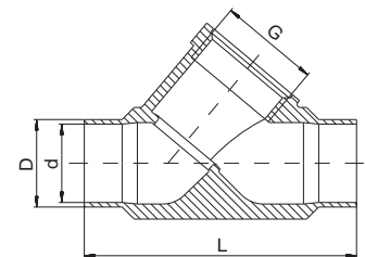
Anschweißenden DIN 11850-2 "M" / welded connection DIN 11850-2 "M"
