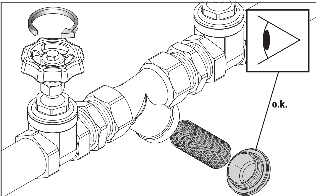
Abb. 5.6 - Schmutzfänger, Reinigen des Siebeinsatzes (Abbildung zeigt Art. BG100025). Option: Absperrschieber TC101025, Doppelnippel A111010
