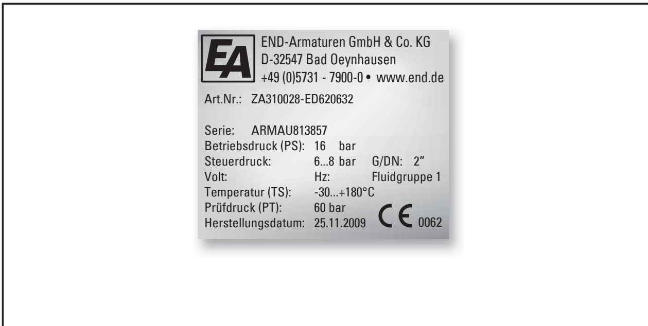
Abb. 4.1 - Typenschild
