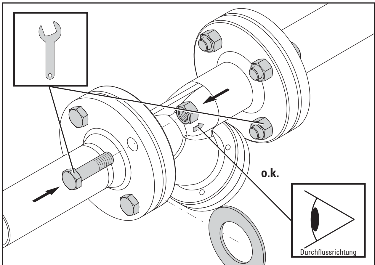
Abb. 5.5 - Schmutzfänger, Montage mit Flanschanschluss (Abbildung zeigt Art. KU3000xx)
