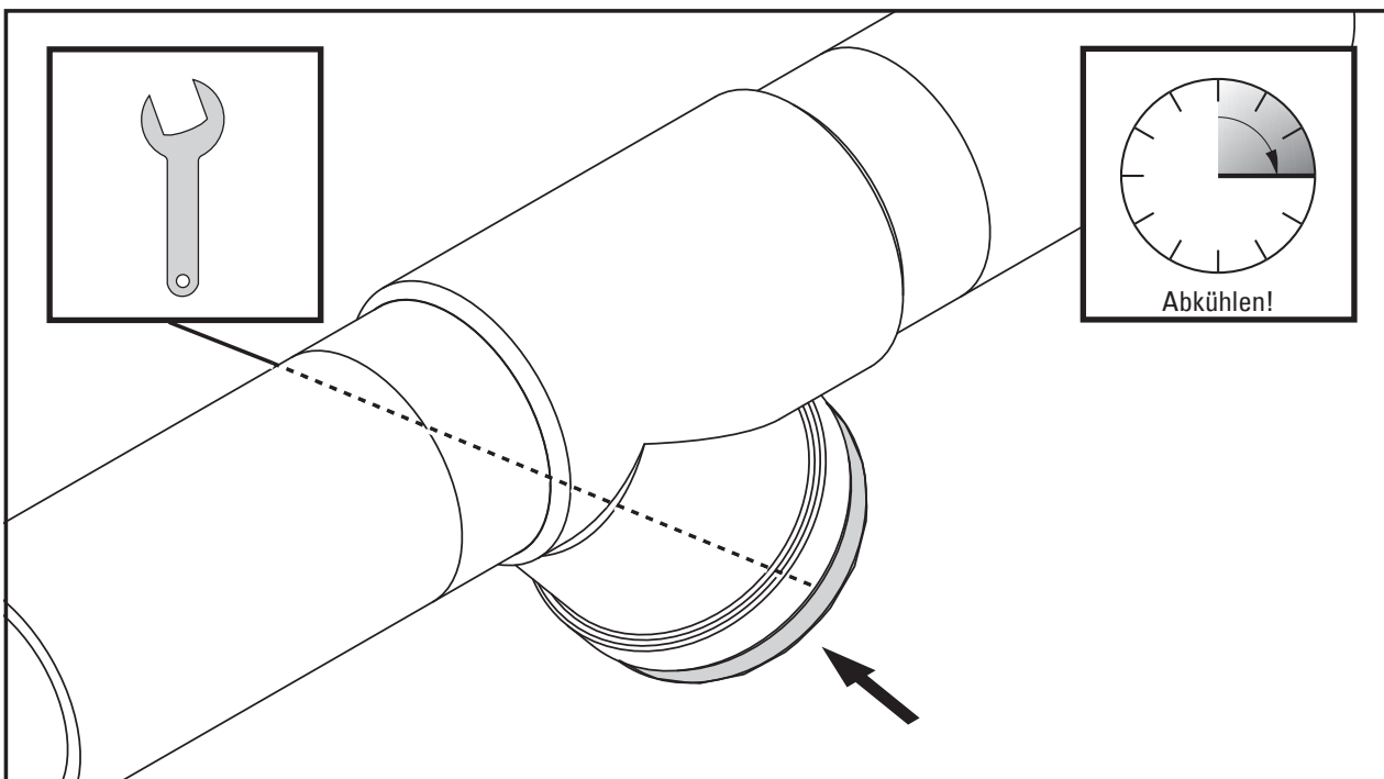
Abb. 5.4 - Schmutzfänger, Montage des Ventiloberteils (Abbildung zeigt Art. EA310064)
